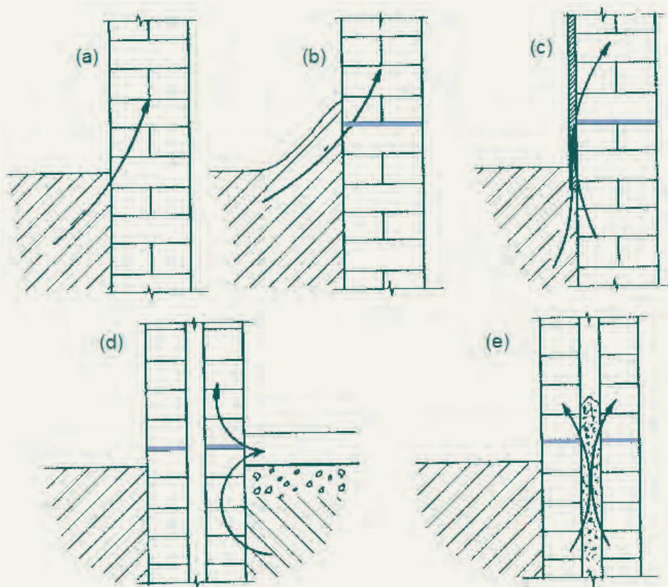
Figura 23 – Umidade ascendente em parede: (a) terra encostada na parede; (b) terra acima da impermeabilização; (c) transmissão pelo revestimento; (d) transmissão pelo contrapiso; (e) transmissão por entulho depositado no vão de parede dupla
