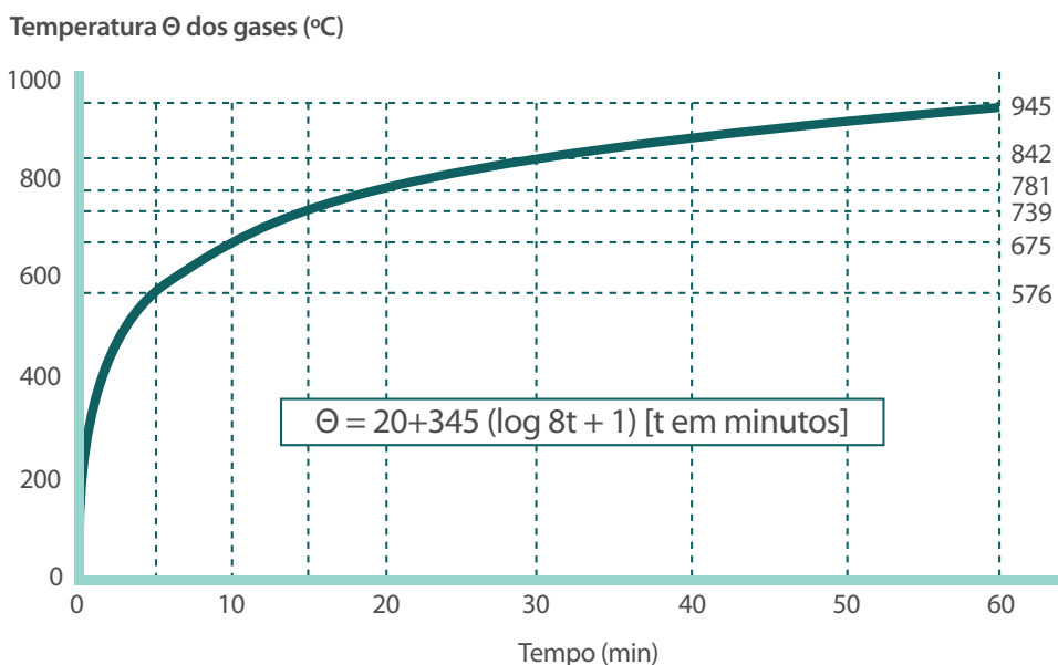
Figura 8 - Curva de crescimento da temperatura e forno de resistência ao fogo (Fonte: IPT).
