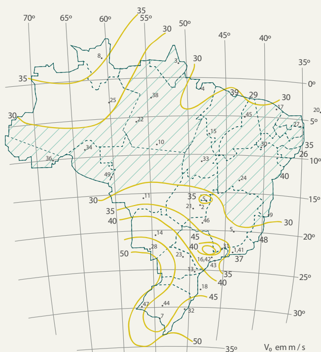
Figura 7 – Mapa de isopletas do vento no Brasil (Fonte ABNT NBR 6123)
